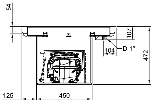
Lato posteriore
